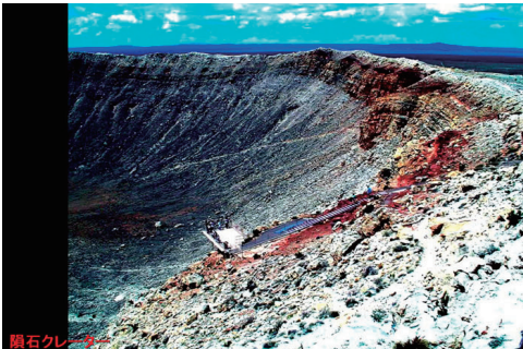
隕石クレーター
