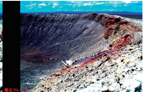
隕石クレーター
